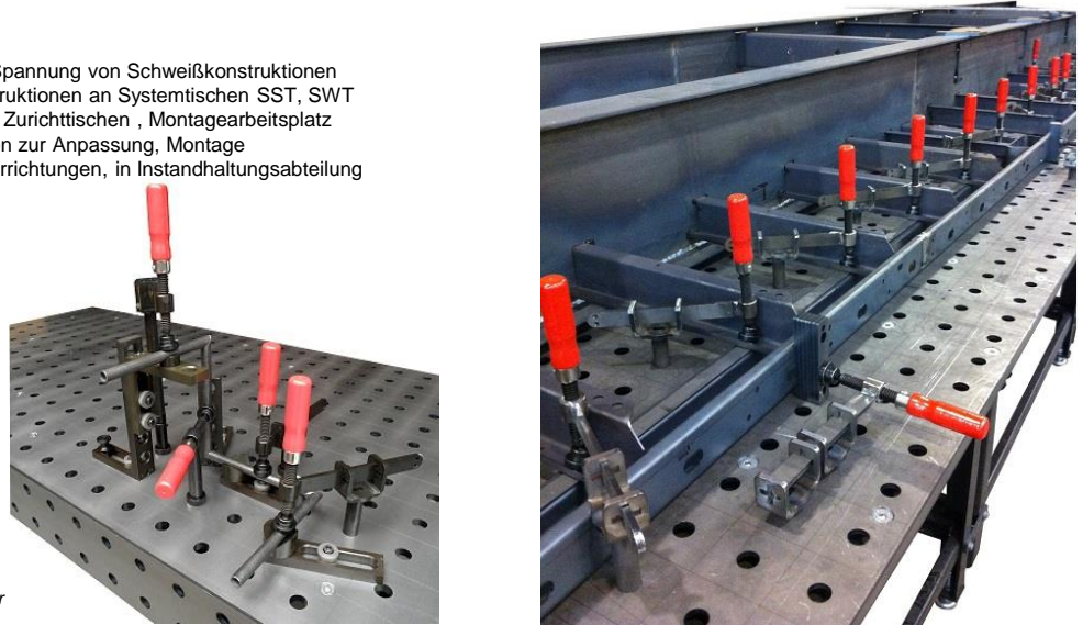
Bilder: Anwendungsbeispiel Spanner
